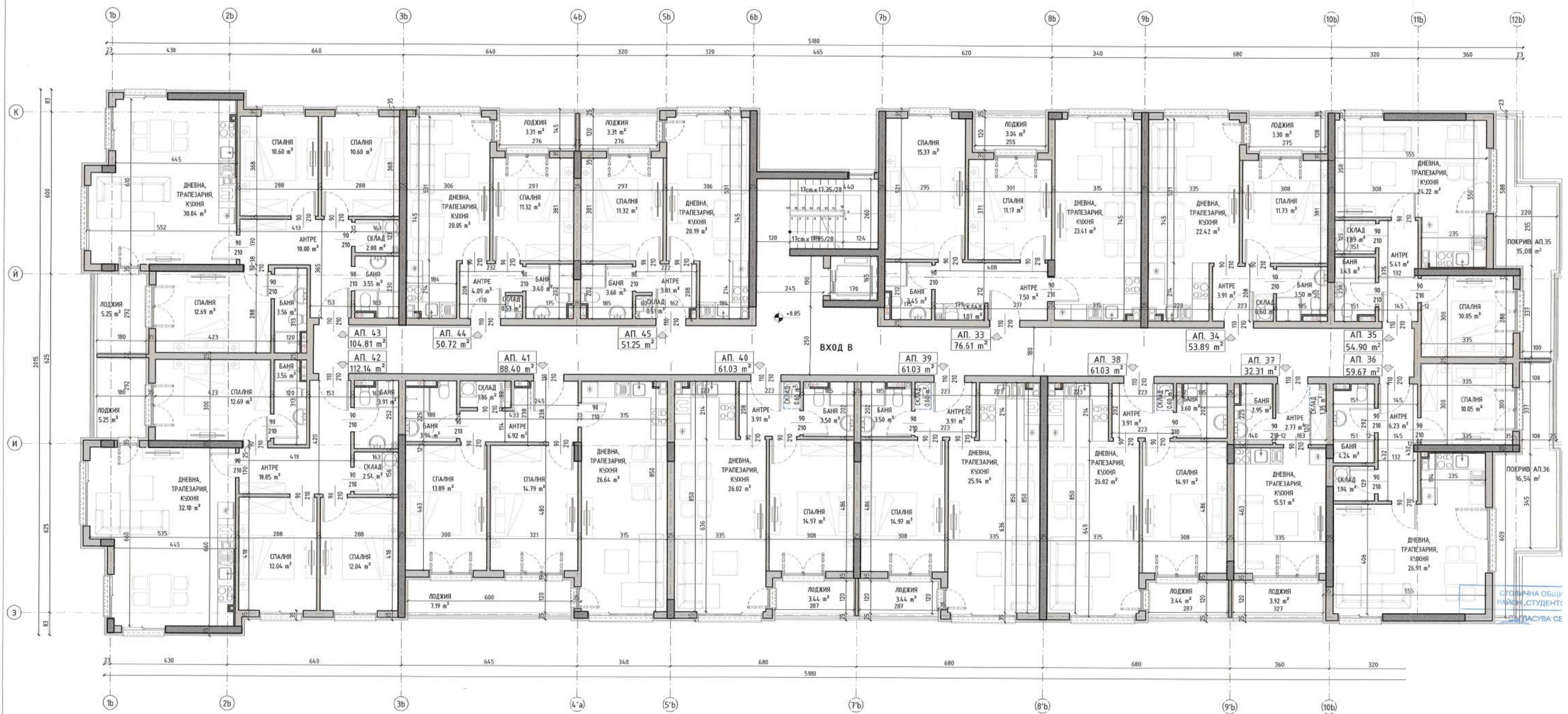
РАЗПРЕДЕЛЕНИЕ КОТА +8.85
