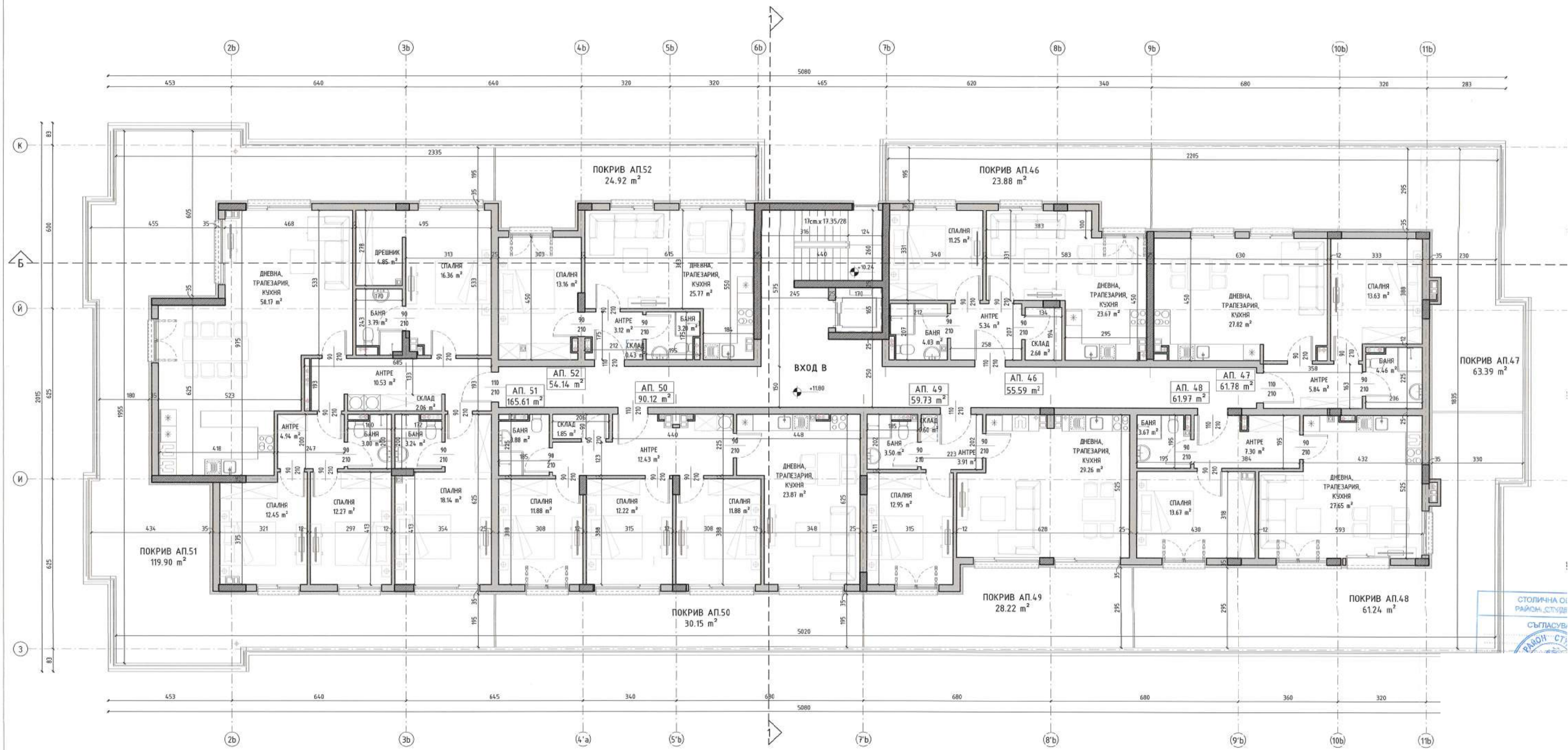
РАЗПРЕДЕЛЕНИЕ КОТА +11.80
